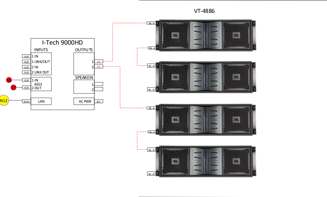
FLOWN CENTER FILL ARRAY
